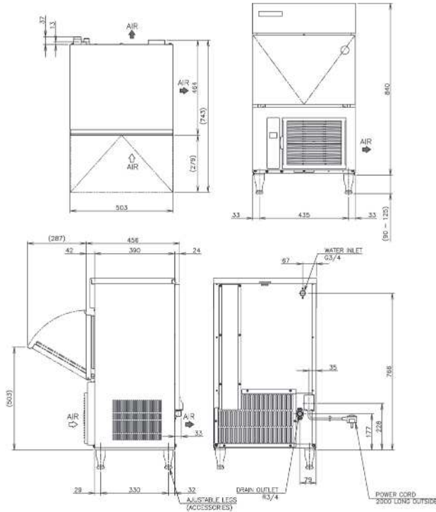
IM-45NE-HC
